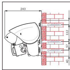
Wandkonsole
