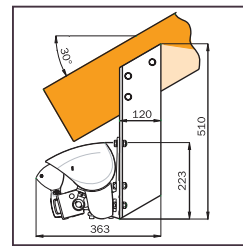
Konsolenplatte
